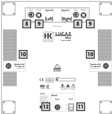
L.U.C.A.S MAX - Bedienfeld Rückseite
